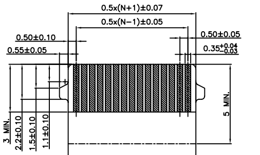
RECOMMENDED FPC DIM.
